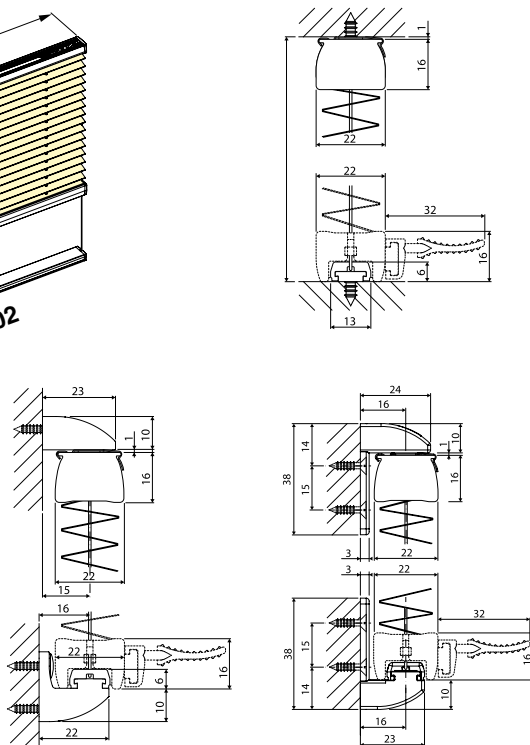
Стеновой кронштейн Comfort
