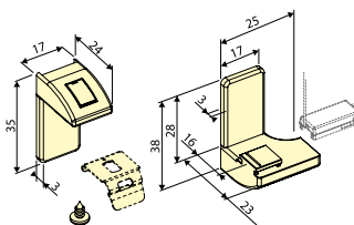
Стеновой кронштейн Comfort
