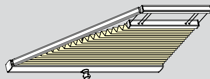
Штора-плиссе — односторонняя трапеция с управлением «крэнк» для наклонного треугольного окна
