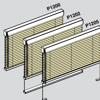
Штора-плиссе с цепочным управлением
