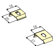
Потолочный замок
