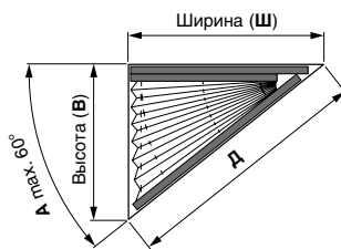
Тип P1141/P1241/P1341
