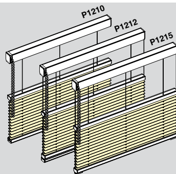
Штора-плиссе с цепочным управлением (подъем шторы снизу вверх)
