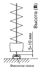
Высота (В) 5-10 мм
