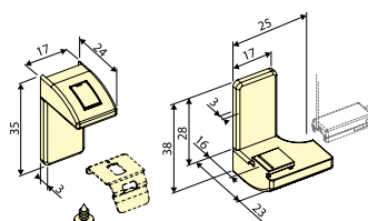
Стеновой кронштейн Comfort
