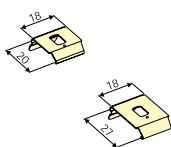
Потолочный замок
