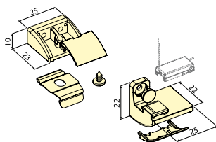
Оконный кронштейн Comfort
