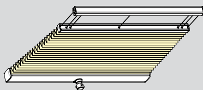
Штора-плиссе трапецевидной формы с управлением «крэнк» для наклонного окна
