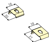
Потолочный замок
