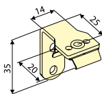
Стеновой кронштейн
