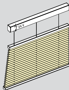
Штора-плиссе — односторонняя трапеция с электроприводом
