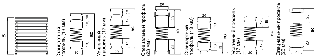
Высота плиссе (В)
