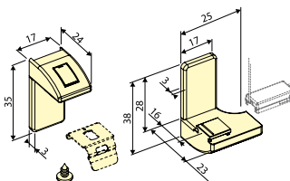
Стеновой кронштейн Comfort
