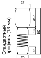
Размер плиссе в собранном виде (BC) 65-69 мм 69-76 мм 72-83 мм 76-90 мм
