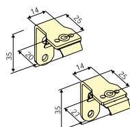
Стеновой кронштейн
