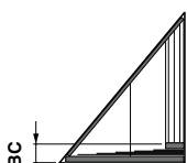
Размер плиссе в собранном виде (BC)
