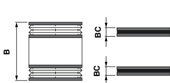
Высота плиссе (В)
